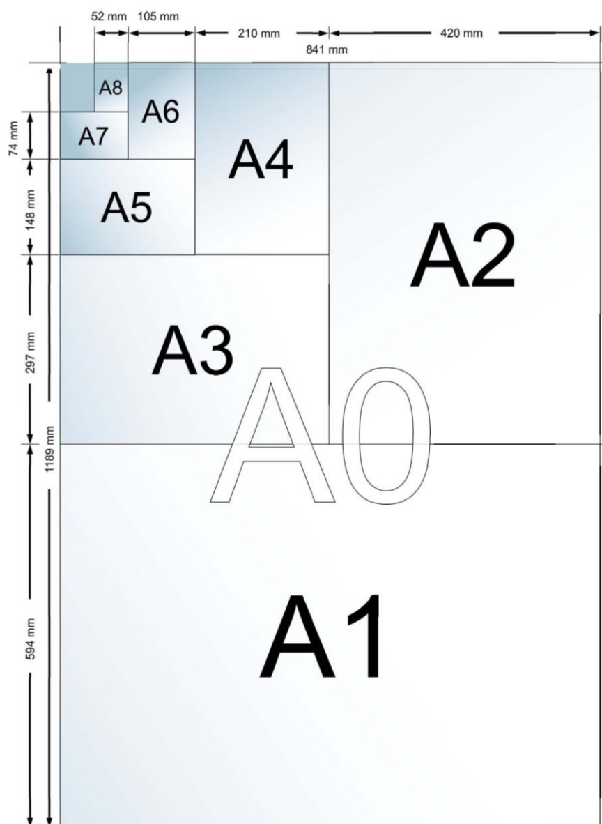
Slika 20: Standardni formati papirja vrste A.
