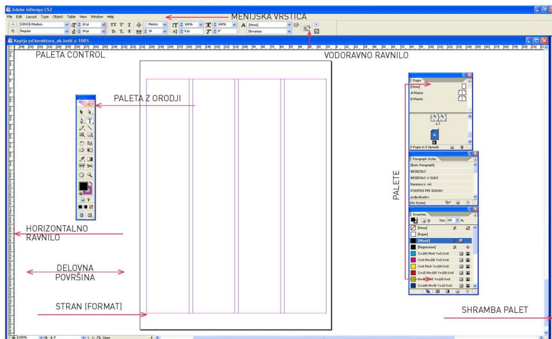
Slika 1: Programsko okno.
